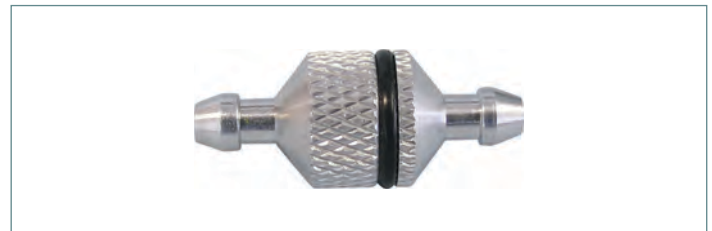
Filtro per carburante Filtre de carburateur Cod. | Réf. 17 7550
