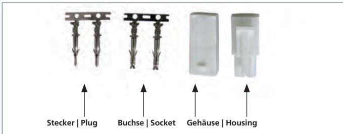
Stecker | Plug
